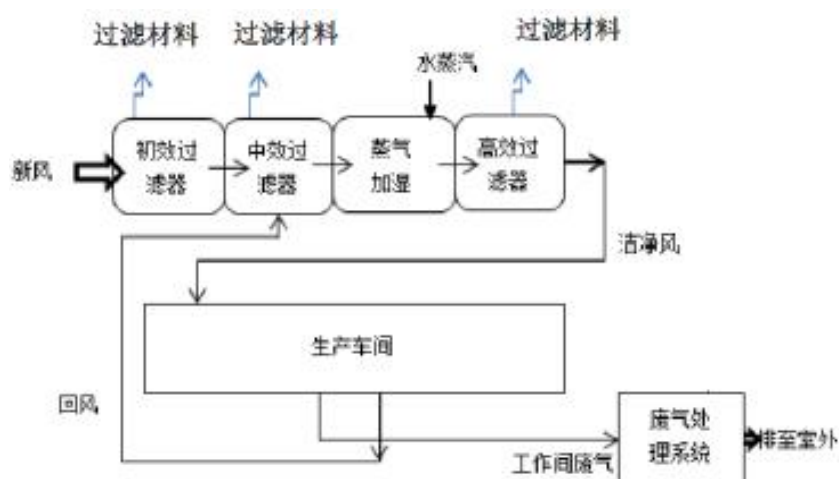
图 3.2-1 空气净化系统空气处理流程
