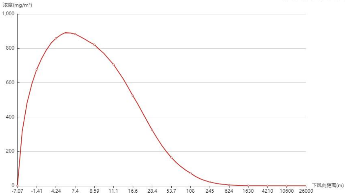
图 6.7-4 常见气象下盐酸泄漏下风向浓度变化曲线
