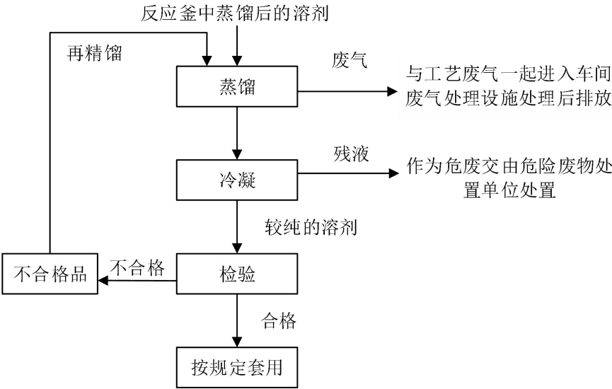
图 3.4-1 溶剂回收系统工艺流程
