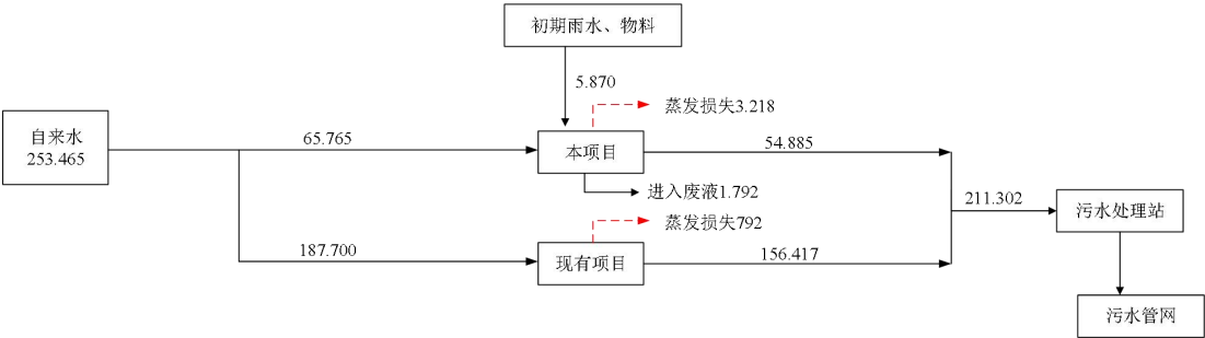
图 3.4-3 项目建成后全厂水平衡图 (单位 \text{t}/\text{d} )
