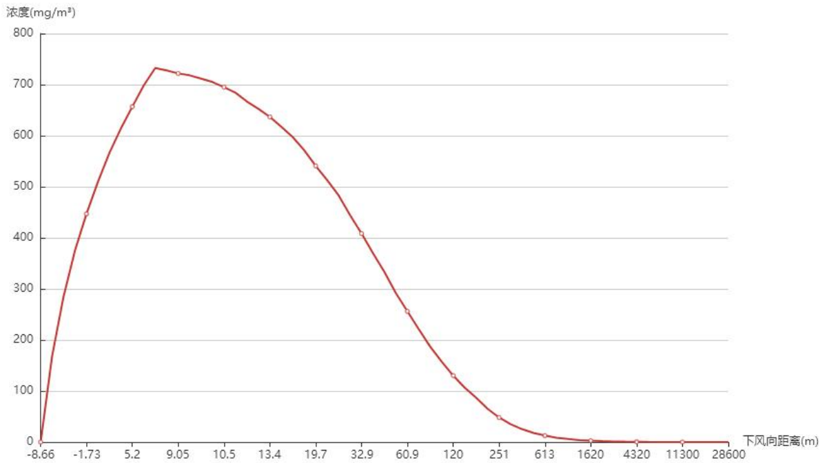
图 6.7-29 最不利气象下乙醇泄漏超过阈值的最大轮廓图
