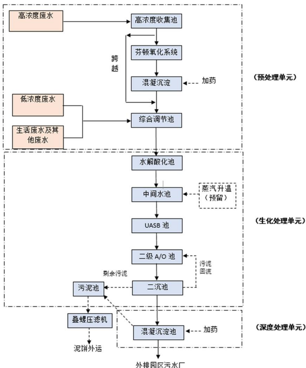
图 7.2-2 2#污水处理站工艺流程示意图
