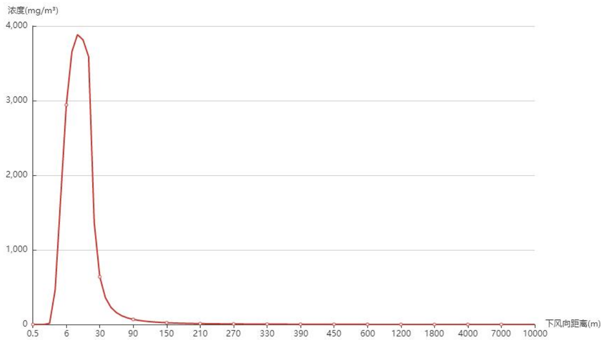
图 6.7-22 最不利气象下丙酮泄漏下风向浓度变化曲线
