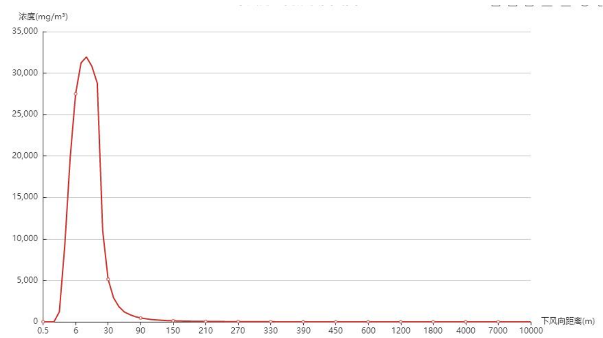
图 6.7-8 常见气象下氨水泄漏下风向浓度变化曲线
