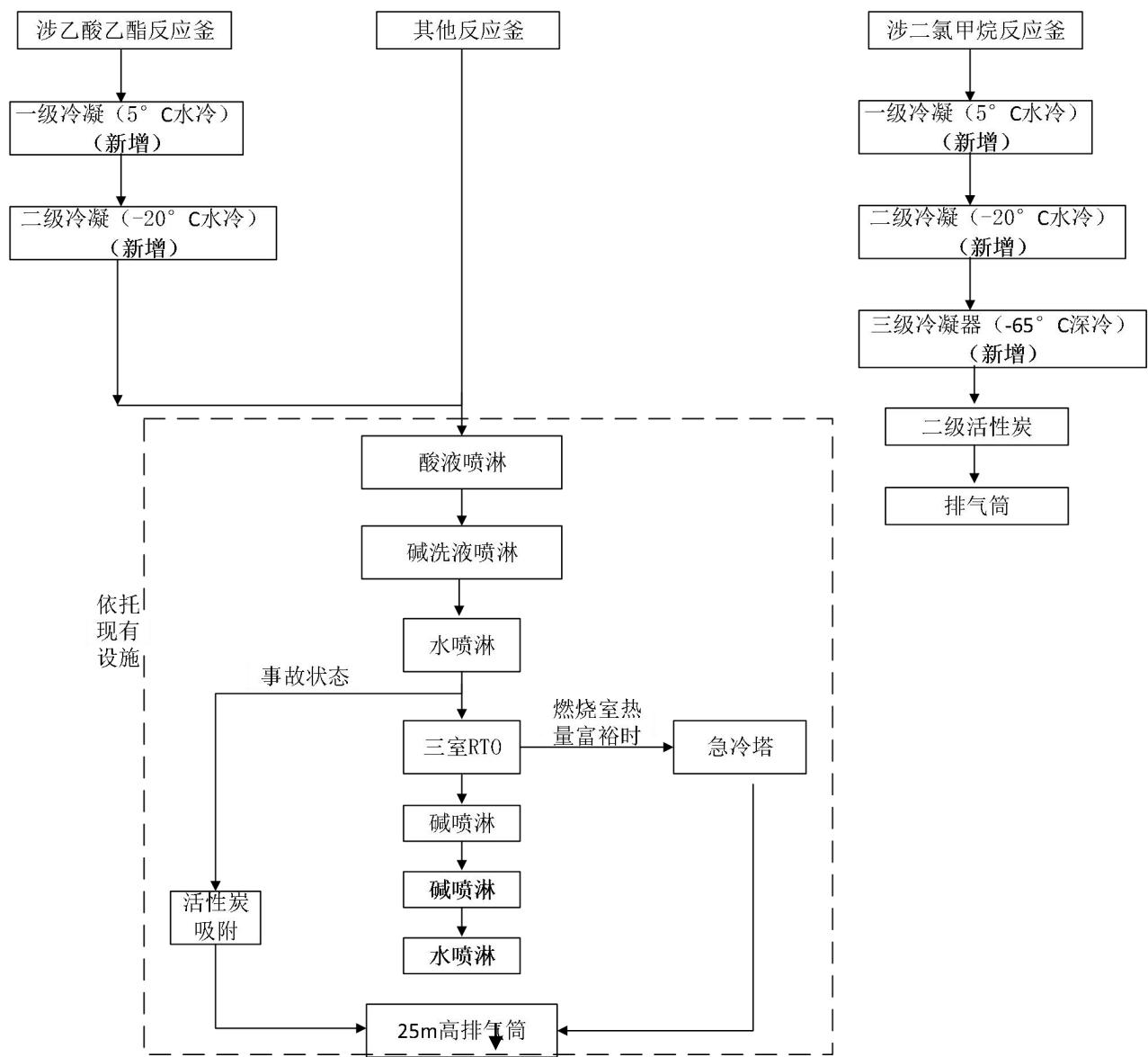
图 3.4-2 项目车间工艺废气治理设施流程图
